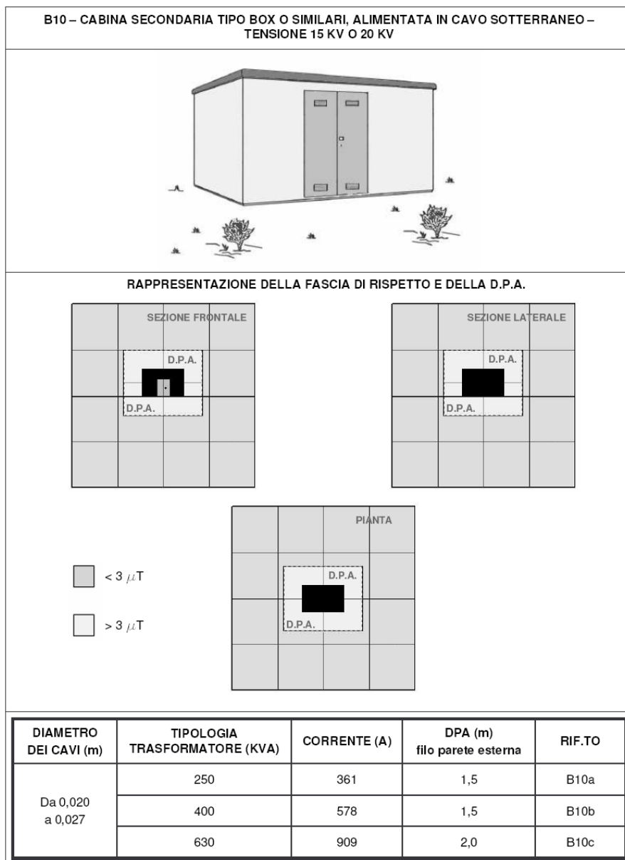
Figura 2 - cabina secondaria
